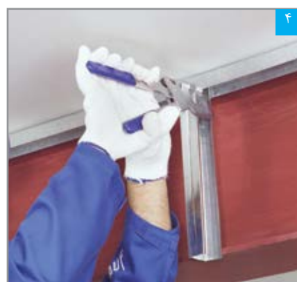
اتصال سازه های قائم به سازه فوقانی (با استفاده از پانچ)
