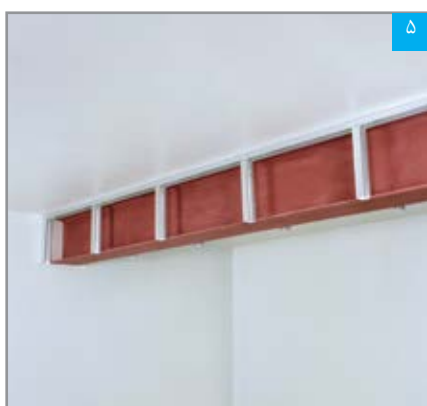
سازه‌های فوقانی و قائم تکمیل شده
