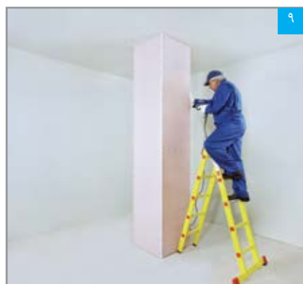
۹ تکمیل پوشش کاری لایه اول
