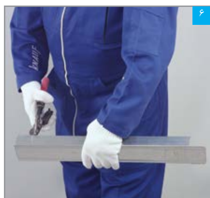
۶ برش سازه پشت بند درز (به صورت زیانه)
