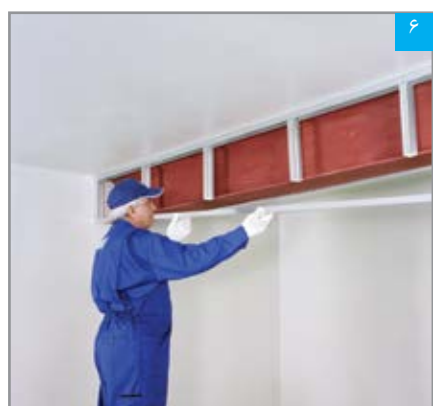
استقرار سازه تحتانی
