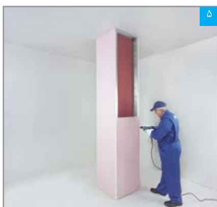
۵ اجرای پنل‌های لایه اول
