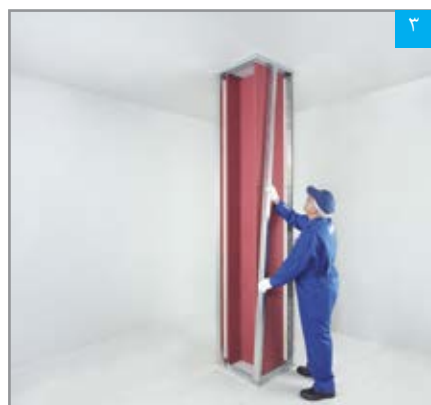
۳ استقرار استاده‌ها در رانتهای کف و سقف
