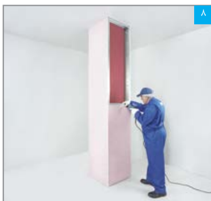
۸ ایجاد اتصال میان سازه پشت بند درز و پنل
