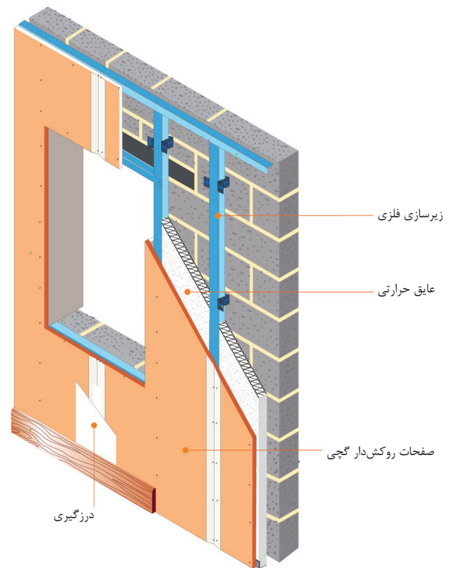
دیوار پوششی با سازه
